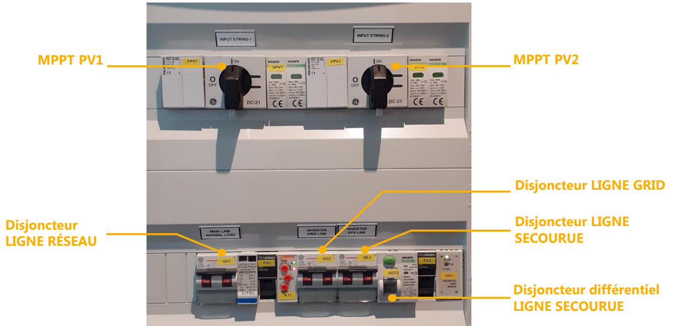
Coffret électrique
