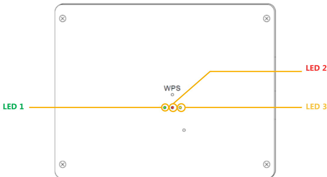
LED d'état de l'armoire H-STORE
